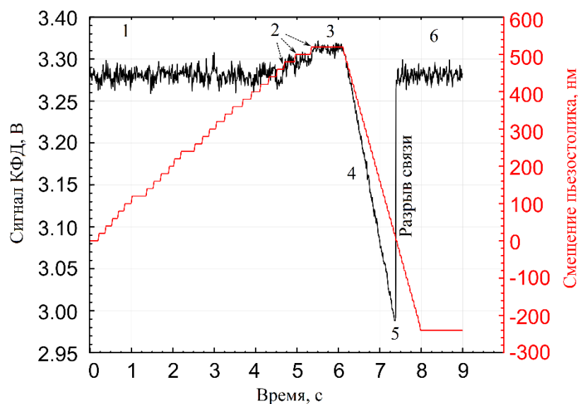
Рис. Хронограмма сигнала квадрантного фотодетектора (V, черный цвет) и соответствующего смещения пьезостолика (нм, красный цвет) для одного из опытов отведения-подведения.
