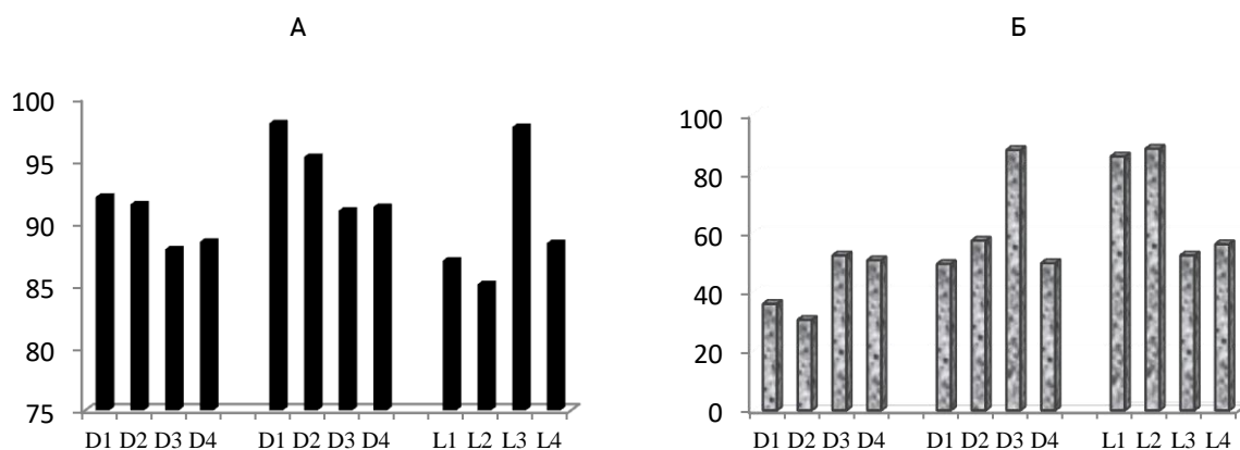
Рис. Степень извлечения радионуклидов (%), А) и доля их необратимой сорбции (%), Б) из водных растворов нитратов урана и тория углеродными наноматериалами детонационного синтеза (D1, D2, D3, D4) и продуктами карбонизации природных и технических лигнинов (L1, L2, L3, L4).
