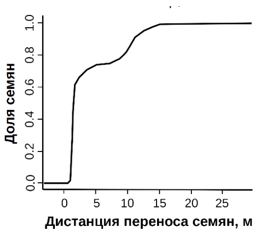
Рис. 1. Моделирование дистанции переноса семян H. sosnowskyi ветром (г. Сыктывкар).
