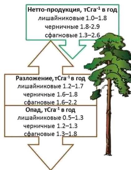
Рис. 2. Потоки углерода в продукционно-деструкционном звене сосняков разных типов.
