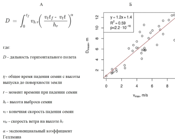
Рис. 2. Градиентная модель анемохорного распространения пропагул H. sosnowskyi (A), зависимость средней дистанции полета искусственных пропагул от скорости ветра (B).
