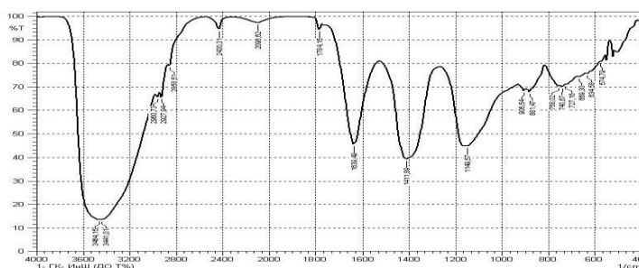
Рис. ИК-спектры препарата гуминовой кислоты, выделенной из угольного шлама.
