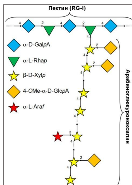
Рис. Структура пектин-арабиноглюкуроноксианового комплекса.
