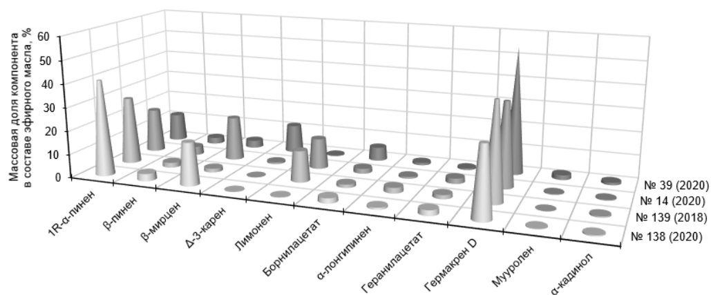
Рис. Изменчивость содержания основных компонентов эфирного масла ( C \geq 0,5 %) в образцах растений S. canadensis , разного географического происхождения. Наименование компонентов приведено в соответствии с данными, отраженными в библиотеке масс-спектров NIST 5.
