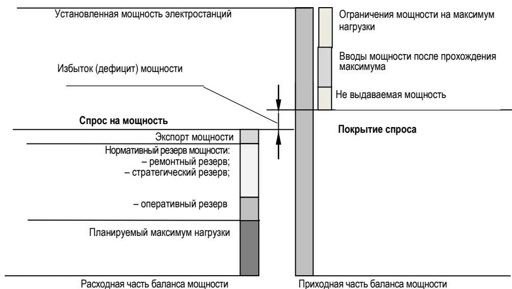
Рис. 1. Структура баланса мощности
