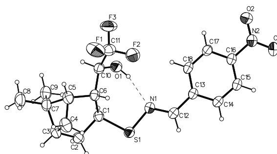
Рис. Структура нитробензилиденсульфенимина 3b на основе 10-гидрокси-10-трифторметилизопинокамфеил тиола по данным PCA.
