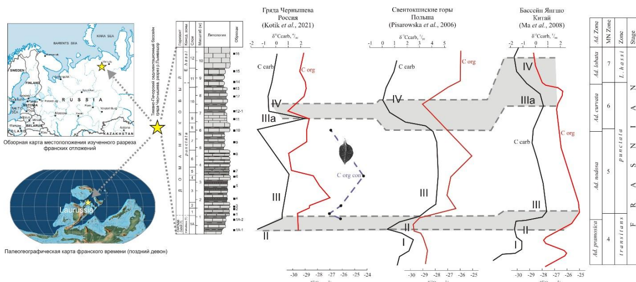
Рис. Сопоставление вариаций \delta^{13}\text{C}_{\text{carb}} и \delta^{13}\text{C}_{\text{org}} в интервале среднефранского глобального изотопного события в разрезах гряды Чернышева, Свѣтокржиских гор (Польша) и бассейна Яншо (Китай).
