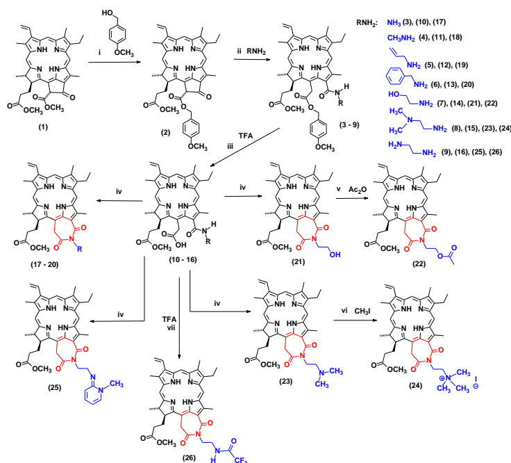
Рис. i: СМПИ, DMAP, толуол, кипячение; ii: \text{CHCl}_3 , ~ 22 °С, 1-5 ч; iii: TFA, ~ 0 °С, 1 ч; iv: СМПИ, DMAP, \text{CH}_2\text{Cl}_2 , кипячение; v: \text{Ac}_2\text{O} , пиридин, 1 ч; vi: \text{CH}_3\text{I} , 2 ч; vii: СМПИ, DMAP, \text{CH}_2\text{Cl}_2 , TFA, кипячение.
