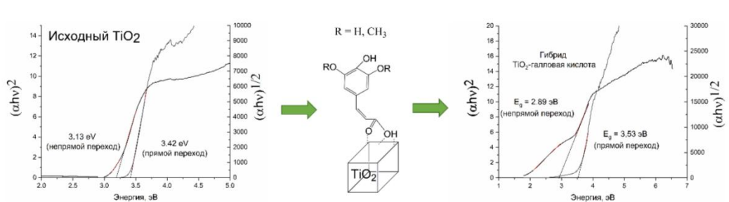
Рис. Кривые Тауца исходного диоксида титана, показывающие сужение ширины запрещенной зоны для не прямых переходов, после его модификации фенольными молекулами.
