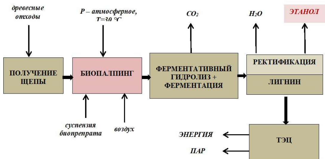
Рис. Схема переработки лиственной древесины с использованием технологии биопалпинга
