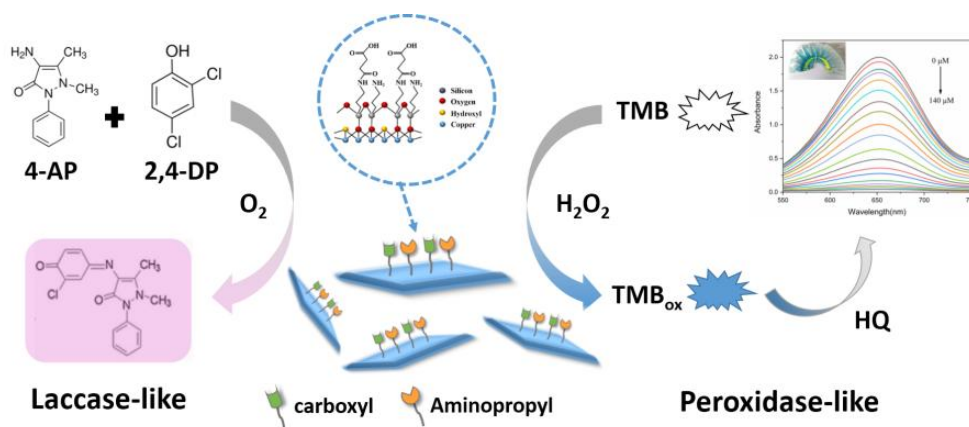
Рис. Схема синтеза аминопропил-функционализированного медьсодержащего органофиллосиликата
