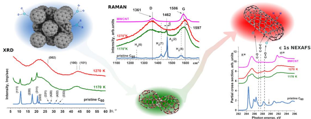
Рис. Модификация фуллерита C 60 в результате HIP-обработки по данным рентгеновской дифрактометрии, рамановской и рентгеновской спектроскопии.
