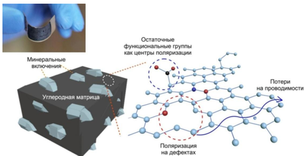
Рис. Ультратонкие гибкие шунгитовые пластинки и ключевые механизмы взаимодействия излучения с шунгитовым веществом
